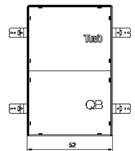
Ingombri predisposizione nuova QB ad incasso
