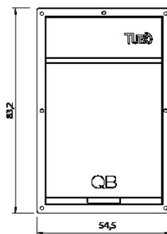
Ingombri nuova QB ad incasso completa
